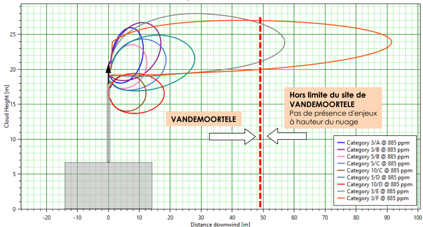
Scénario 13 - Fuite liquide installation à l'arrêt avec pression BP élevée à +1°C (sat) avec vannes de sécurité Rejet Extracteur SDM1 (SEI)
