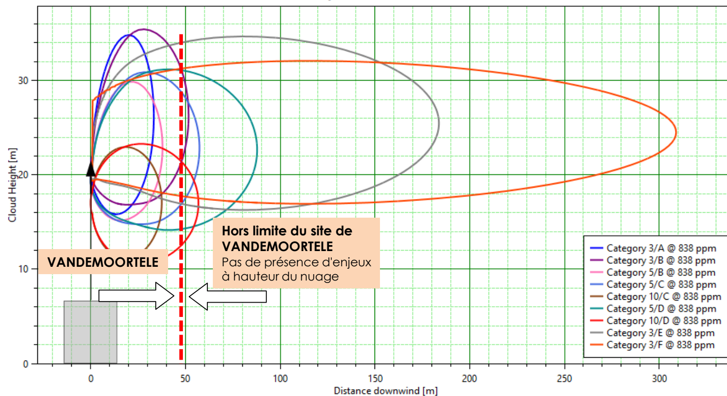
Scénario 13 - Fuite liquide installation à l'arrêt avec pression BP élevée à +1°C (sat) sans vannes de sécurité Rejet Extracteur SDM1 (SEI)
